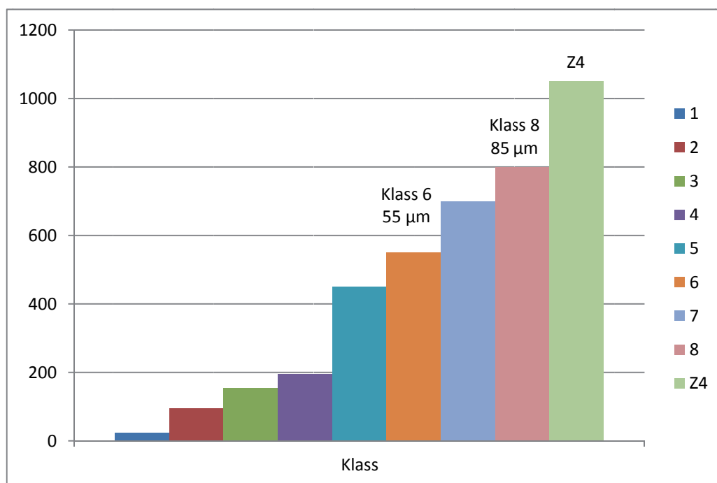
Timer eksponert i saltspraytest
