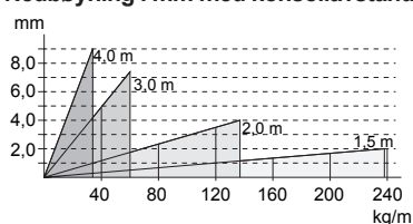
Nedbøyning i mm med konsollavstand 1,54 m.
