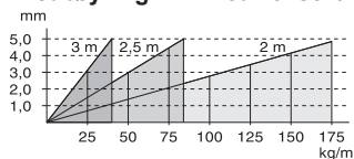
Nedbøyning i mm ved konsollavstand 2-3 m.
