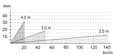
Nedbøyning i mm med konsollavstand 2-4 m.
